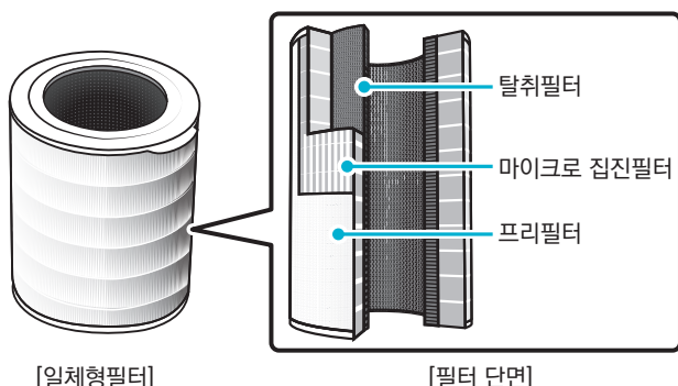
[일체형필터]
